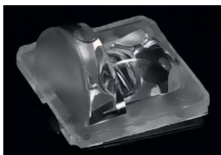
Рис. 7. Внешний вид и КСС линзы CS14713_HB-2X2MX-W
