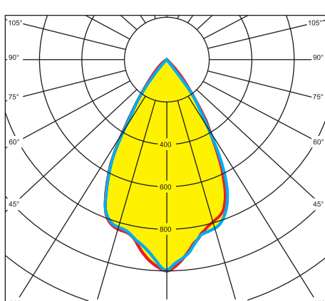
Рис. 7. Внешний вид и КСС линзы CS14713_HB-2X2MX-W
