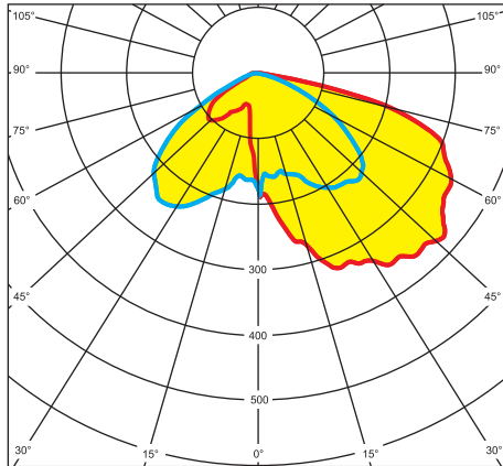
Рис. 9. Внешний вид и КСС линзы F14563_JENNY-T4
